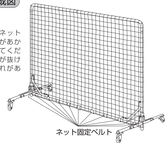
完成図
