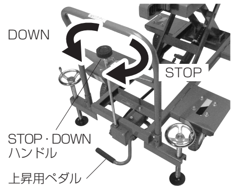
【図-5】 型式 COU、COR
