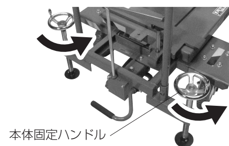
【図-10】 型式 COU、COR
