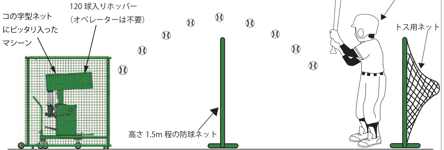
(型式 ARMLHタイプ) 例—3 単独打席にて使用
